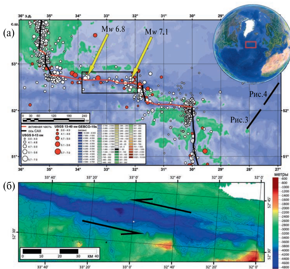
Рис. 1. Район двойного трансформного разлома Чарли Гиббс. (а) — сейсмичность по данным [1, 2], рельеф дна по данным [3], положения разрезов рис. 3 и рис. 4, на врезке общее положение района исследований в Северной Атлантике, прямоугольником показано положение планшета рис. 1 б с детальным рельефом; (б) — левосдвиговая впадина пулл-апарт по данным многолучевой батиметрии 50-го рейса НИС “Академик Николай Страхов” (ГИН РАН, 2020) на оси северного трансформного трога.
