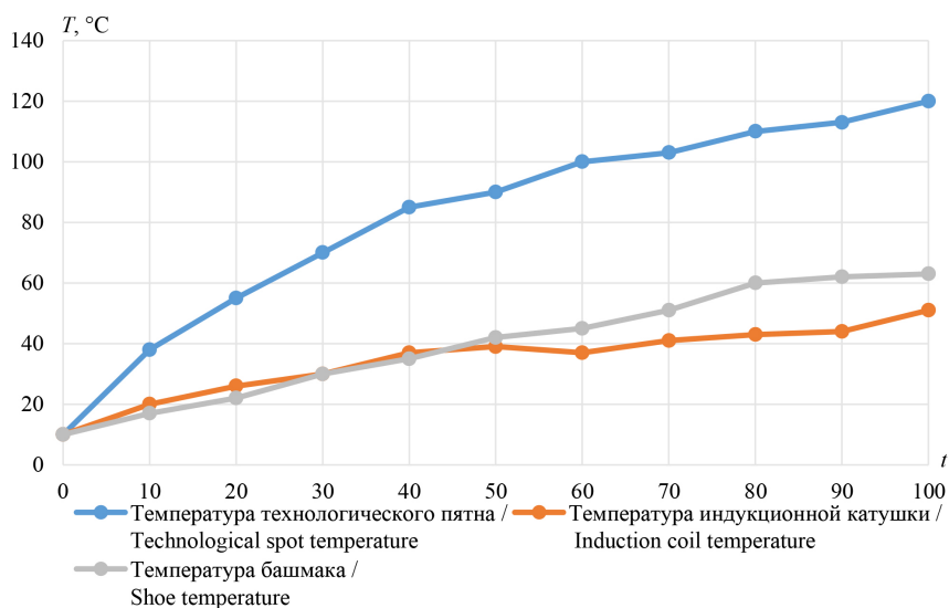
Р и с. 4. Зависимость температуры нагрева элементов устройства от времени
