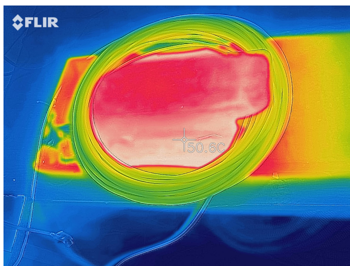
Р и с. 3. Тепловизионный снимок индукционного нагревателя
