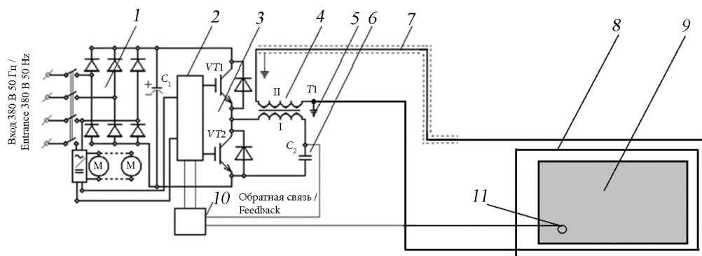
Р и с. 2. Электрическая схема прямого точечного индукционного нагрева повышенной частотой подушки скольжения башмака стрелочного перевода:
