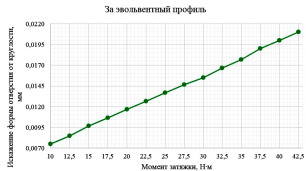
Рис. 3. График зависимости искажений формы отверстия от круглости \Delta r_{s3i} в зависимости от момента затяжки M_{s3i} (закрепление за эвольвентный профиль) Fig. 3. Dependence diagram of hole shape distortion from \Delta r_{s3i} roundness as a function of tightening torque M_{s3i} (fixing by involute)
