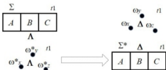
Рис. 3. Схема квантовой телепортации
