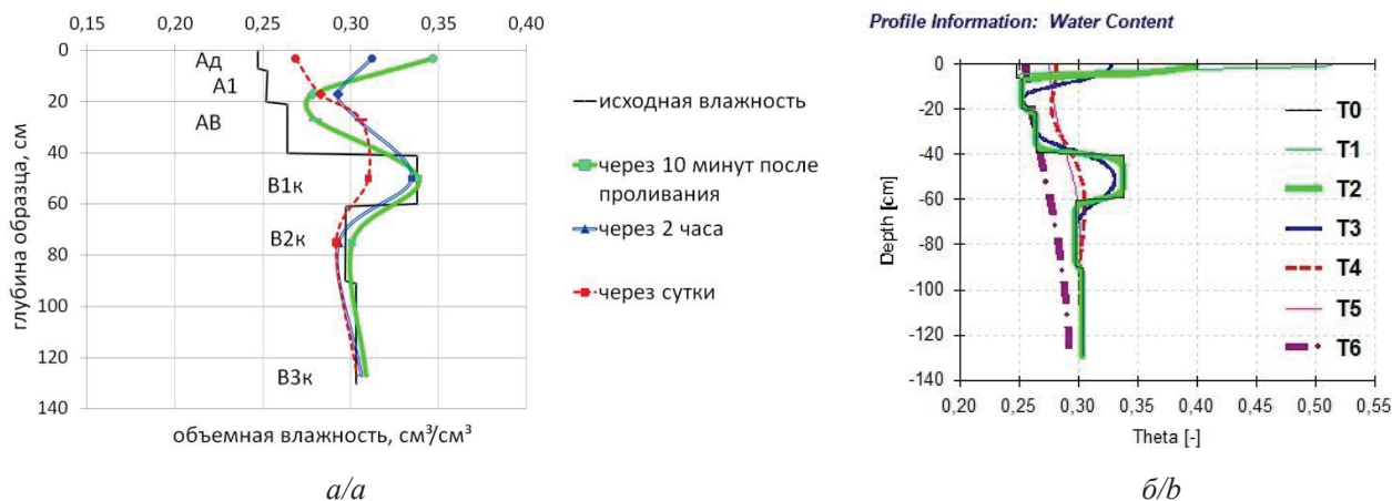
Рис. 6. Профильное распределение влаги в черноземе выщелоченном яблоневого сада опытной станции «Горно-Алтайское» после дождя (эквивалентно выпадению 20 мм осадков): измеренные содержания (а) и смоделированные в Hydrus-1D значения (б)
