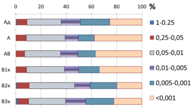
Рис. 2. Диаграмма распределения гранулометрических фракций (по [9]) с глубиной в профиле чернозема выщелоченного под яблоневым садом опытной станции «Горно-Алтайское»
