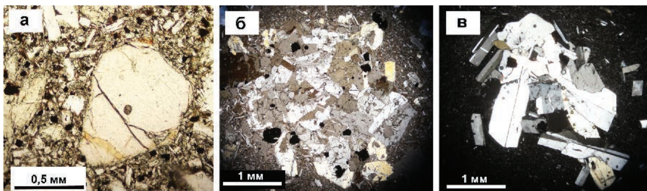
Рис. 2. Вкрапленники плагиоклаза в базальте (а), андезите (б) и даците (в). Проходящий свет; фото б, в – с поляризатором.
