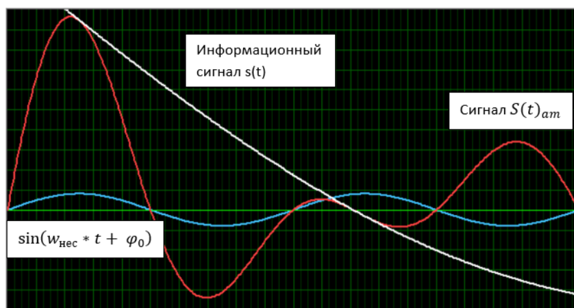
Рисунок 6.б) – Информационный сигнал за один период несущего колебания изменяет свой знак однократно, эта смена не совпадает со сменой знака несущего колебания: у результирующего колебания обнаружены два уменьшенных полупериода – до и после перехода огибающей через ось времени
