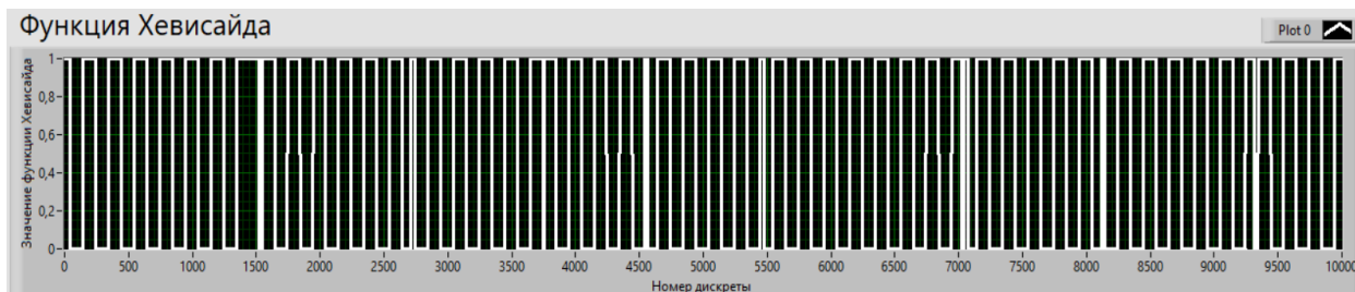
Рисунок 9 – Сигнал, получаемый с выхода блока функции Хевисайда: длительность прямоугольных импульсов численно равна длительности положительных полупериодов принимаемого колебания
