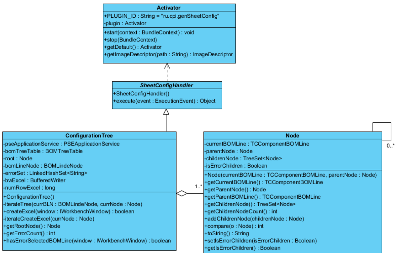
Рис. 3. Диаграмма классов.
