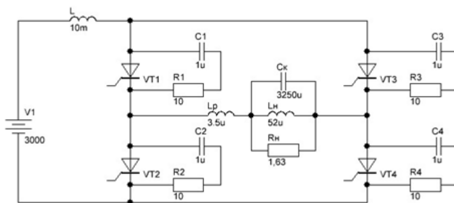
Рис. 1 Упрощенная схема инвертора тока. В каждом плече инвертора – 4 тиристора.
