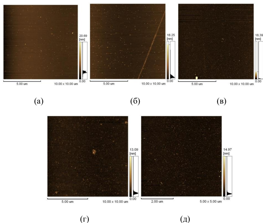
Рис. 2. Изображения СЗМ, полученные при различных температурах процесса: (а) 100 °C, (б) 150 °C, (в) 200 °C, (г) 250 °C, (д) 300 °C.
