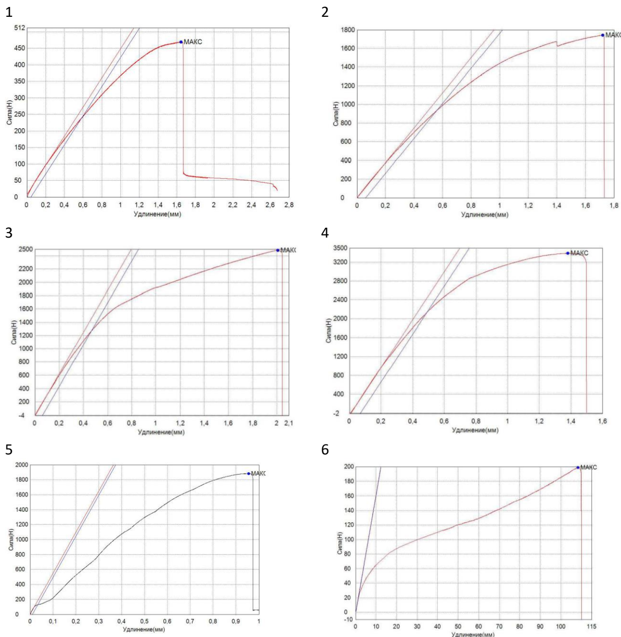
Рис. 1. Диаграммы деформации (номер соответствует образцу полимера).
