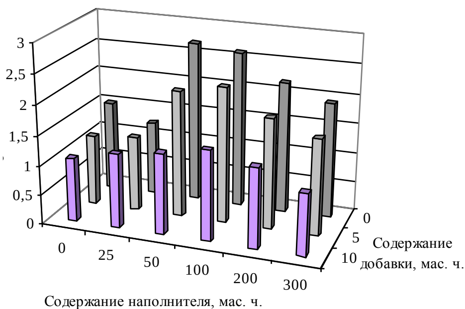
Рис. 4. Зависимость изменения водопоглощения по массе полимерных композитов на основе эпоксидной смолы и аминифенольного отвердителя, наполненных отсеком дробления гранитного щебня от степени наполнения и содержания добавки «Тефлекс».
