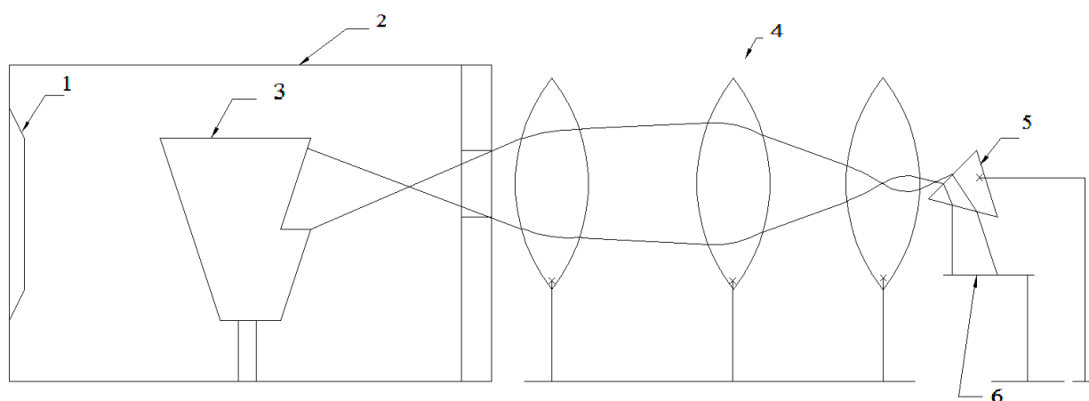
Рис. 3. Технологическая схема организации непрерывного источника ионов на СВЧ плазменных технологиях и фиксации спектров твердых веществ
