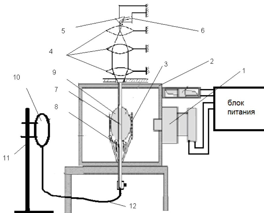
Рис. 4. Технологическая схема организации непрерывного источника ионов на СВЧ плазменных технологиях и фиксации спектров жидких веществ
