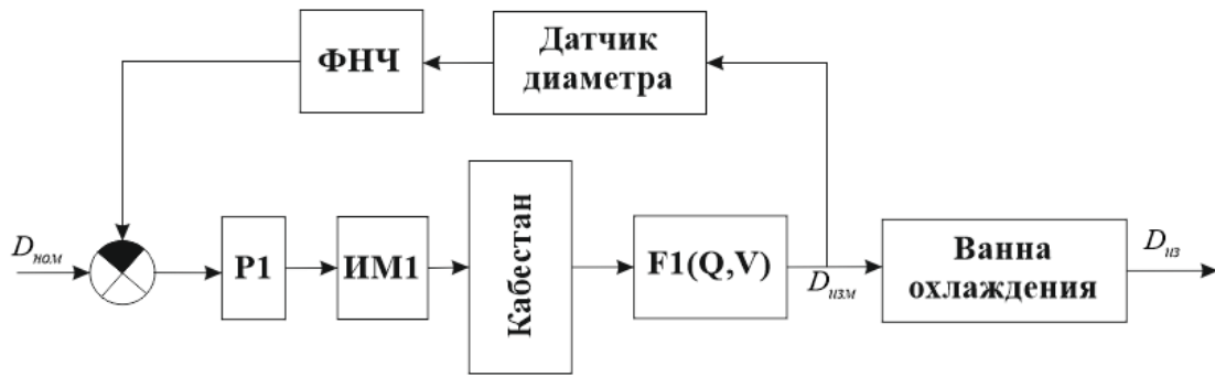
Рис. 2. Функциональная схема управления процессом наложения полимерной изоляции при управлении приводом кабестана: D_{ном} – номинальное значение диаметра изоляции в месте измерения; D_{изм} – диаметр изоляции, измеренный на выходе экструзионной линии; D_{из} – диаметр изоляции, измеренный на выходе ванны охлаждения; P1 – регулятор контура регулирования диаметра; ИМ1 – исполнительный механизм тянущего устройства (привод кабестана); ФНЧ – низкочастотный фильтр; Q – весовая производительность экструдера; V – протяжки кабельной жилы; F1 – аналитическая зависимость, связывающая значения соответствующих параметров.
