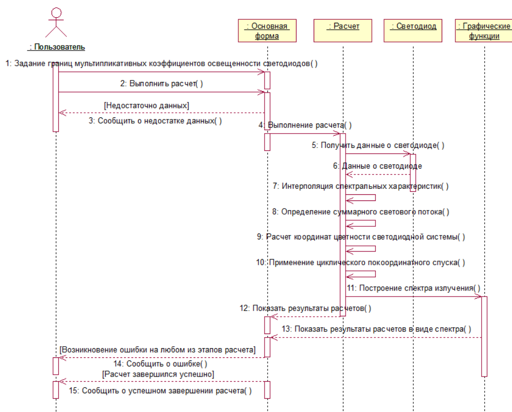
Рис. 1. Диаграмма последовательности для прецедента «Ввод данных».
