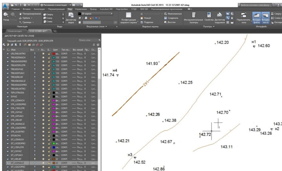
Рис. 3. Фрагмент цифровой модели рельефа на изучаемую территорию.
