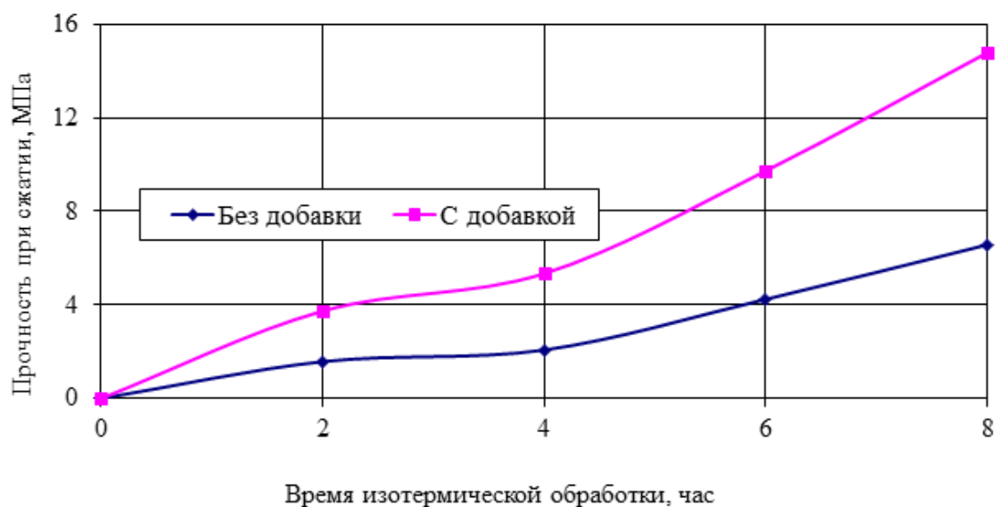
Рис. 2. Влияние продолжительности тепловлажностной обработки цементных композитов на рост их прочности.
