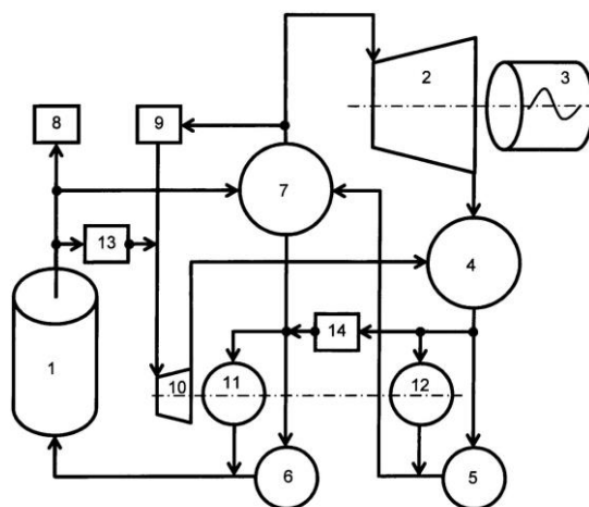
Рис. 4. Схема атомной электрической станции (патент на изобретение RU 2638305 C1 [4]).
