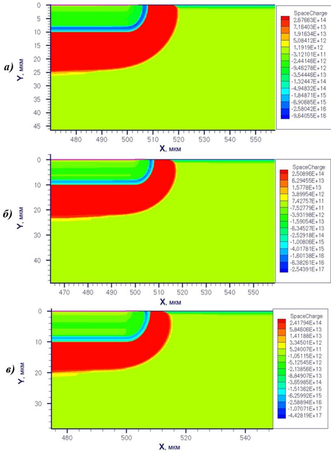
Рис. 3. Распределение ОПЗ для поверхностной концентрации заряда в окисле:
