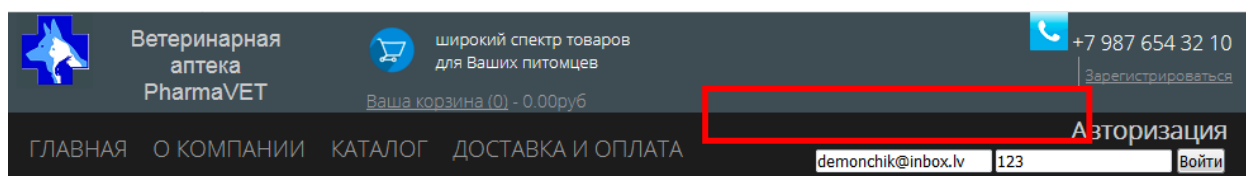
Рис. 7. Форма авторизации.
