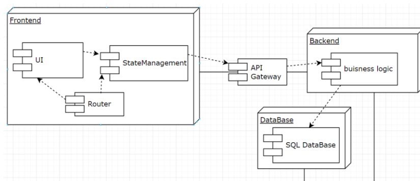
Рис. 6. Диаграмма компонентов.
