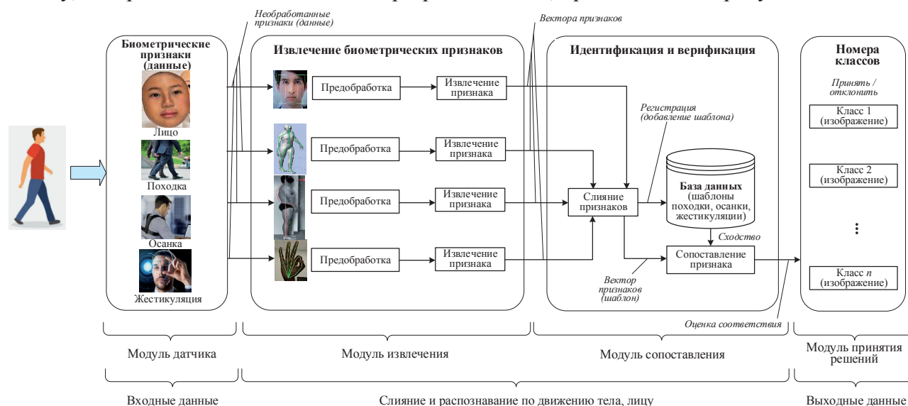
Рисунок 5 – Структурная схема слияния биометрических данных и распознавания нарушителя по движениям тела и лицу
