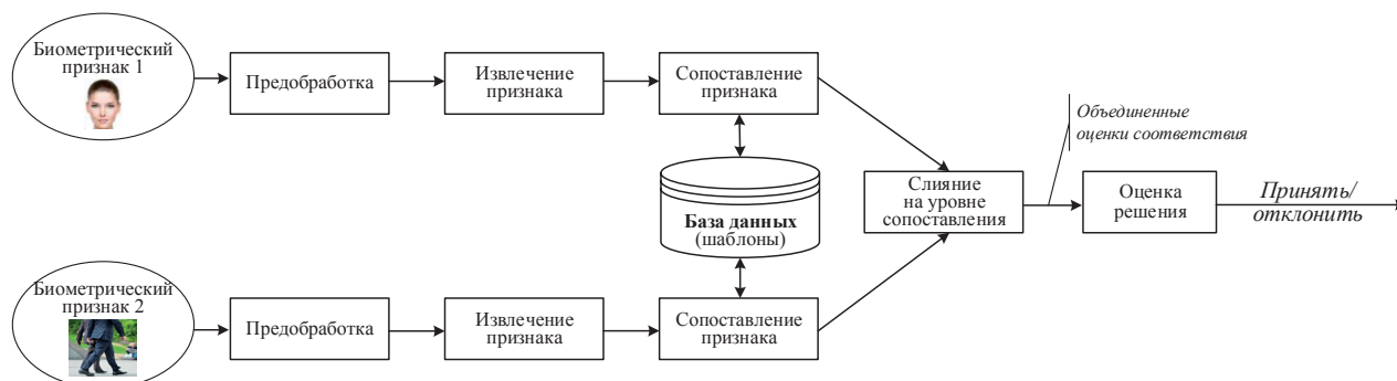
Рисунок 9 – Слияние данных на уровне оценки сопоставления
