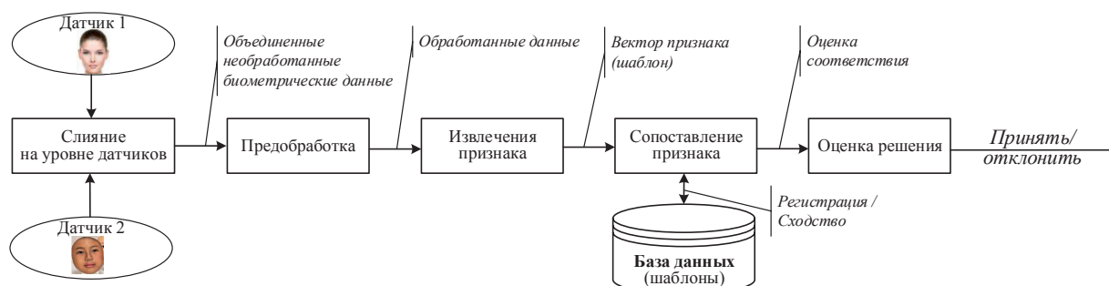
Рисунок 7 – Слияние данных на уровне датчиков
