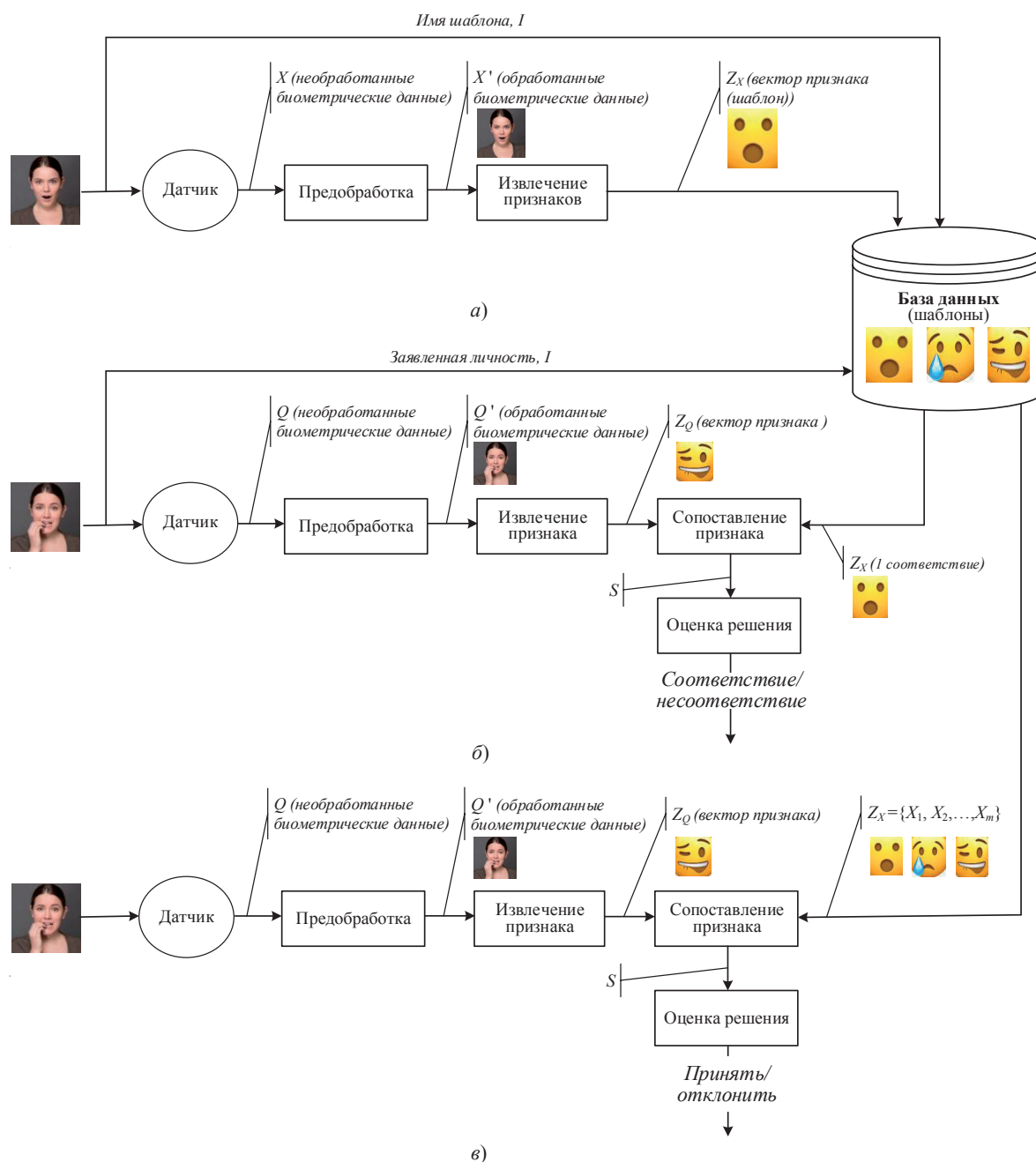
Рисунок 11 – Схемы процесса биометрической аутентификации:
