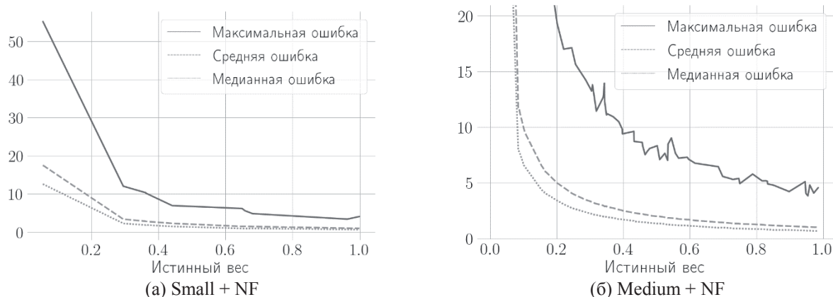
Рисунок 1 – Ошибки источников в зависимости от их истинного веса
