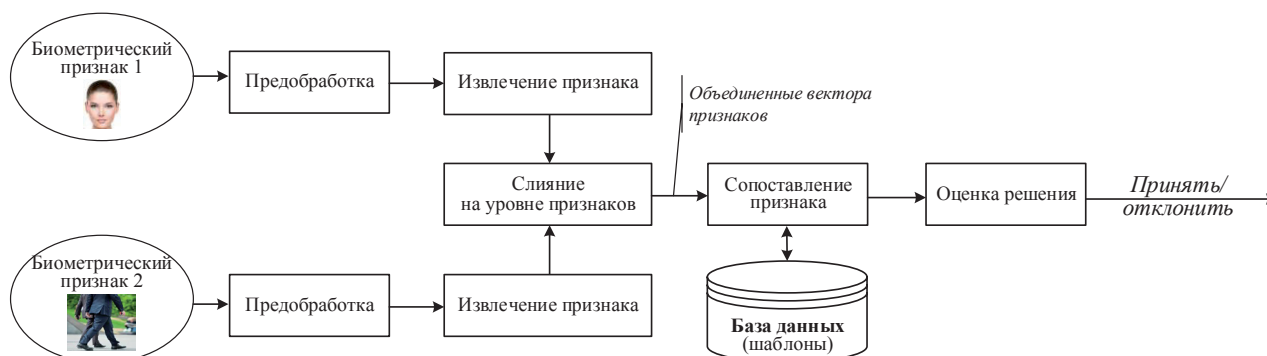
Рисунок 8 – Слияние данных на уровне признаков
