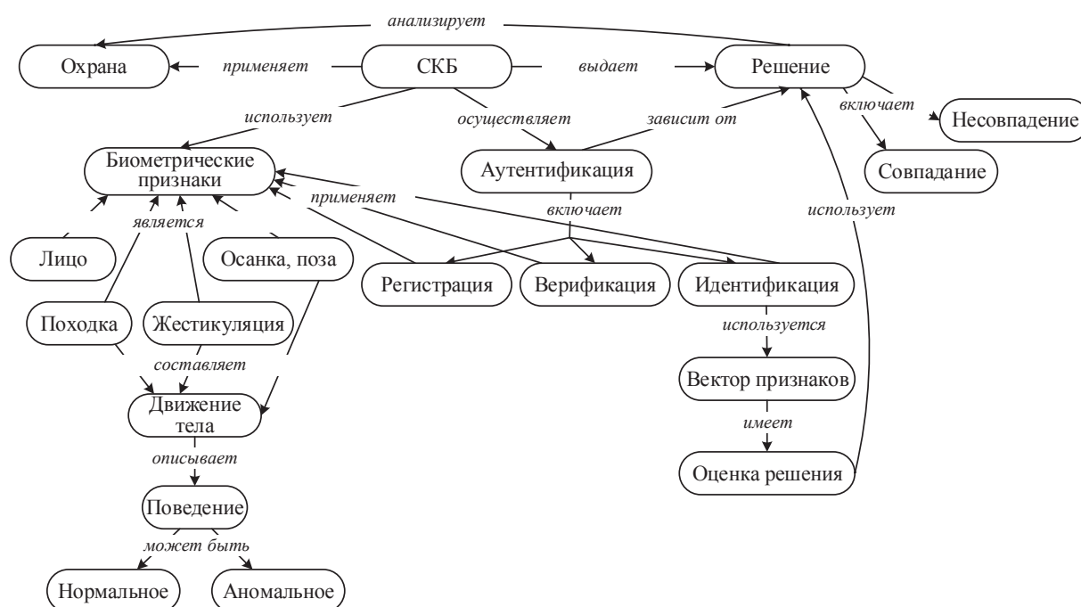
Рисунок 1 – Фрагмент онтологии процесса идентификации нарушителя
