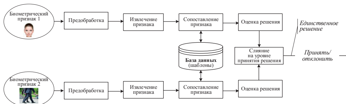
Рисунок 10 – Слияние данных на уровне принятия решения
