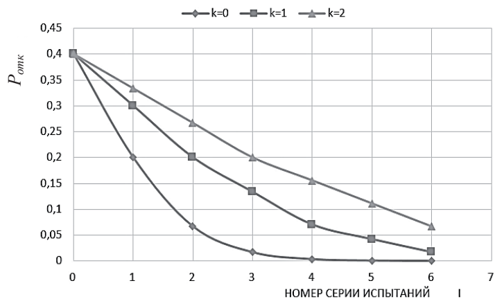
Рисунок 2 - Динамические характеристики интегрального показателя ФБ
