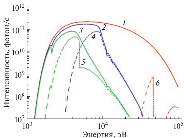
Рис. 2. Расчетная спектральная мощность СИ (в энергетической полосе \Delta E/E = 10^{-3} ) на расстоянии 55 м от точки излучения, приходящаяся на 1 см площади по горизонтали, проинтегрированная по углу в вертикальной плоскости с учетом установленных на пути излучения окон из бериллия и фильтров. Источник излучения: поворотный магнит с напряженностью поля H = 20 кГс; 1 — бериллиевое окно толщиной 200 мкм; 2 — бериллиевое окно толщиной 200 мкм и зеркало с платиновым покрытием, ориентированное под углом 0.5^\circ к горизонтали; 3 — бериллиевое окно толщиной 200 мкм и платиновое зеркало под углом 1^\circ ; 4 — бериллиевое окно 200 мкм, алюминиевый фильтр толщиной 50 мкм и платиновое зеркало под углом 0.5^\circ ; 5 — бериллиевое окно толщиной 200 мкм, титановый фильтр толщиной 10 мкм и платиновое зеркало под углом 1^\circ ; 6 — бериллиевое окно толщиной 200 мкм и селективный фильтр Sm/Eu толщиной 700/200 мкм соответственно.
