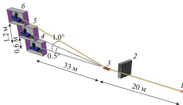
Рис. 1. Блок-схема станции: 1 — источник излучения; 2 — радиационная защита; 3 — плоское зеркало скользящего падения; 4 — модуль прямого пучка; 5 — модуль пучка, отраженного под углом 0.5^\circ ; 6 — модуль пучка, отраженного под углом 1^\circ .
