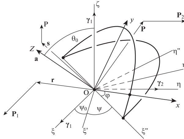
Рис. 1. Геометрическая трактовка прецессий твердого тела.
