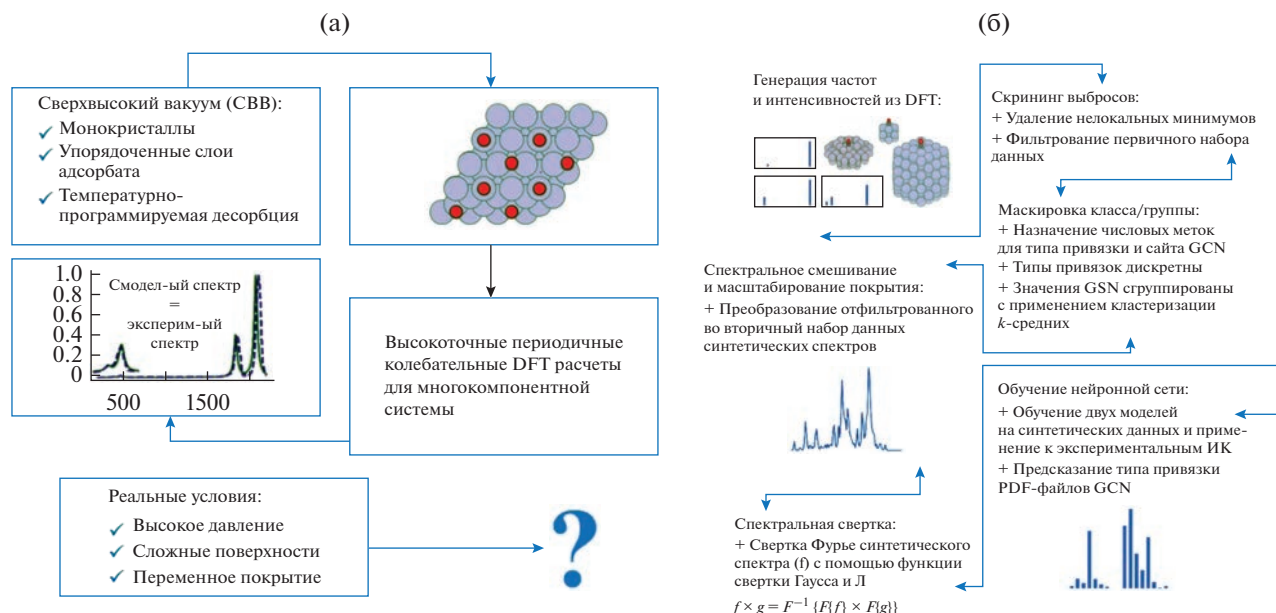
Рис. 12. Подход, объединяющий экспертные знания и спектроскопические данные для устранения “materials gap”. “Materials gap” (a) и соответствующий рабочий процесс для его устранения (б). Адаптировано из [30]. Распространяется на условиях лицензии Creative Commons CC BY license. Adapted from [30]. Distributed under the terms of the Creative Commons CC BY license.
