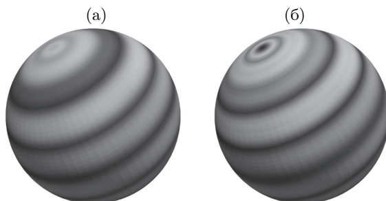
Рис. 1. Модуль функций плотности \phi(x) и \psi(x) .
