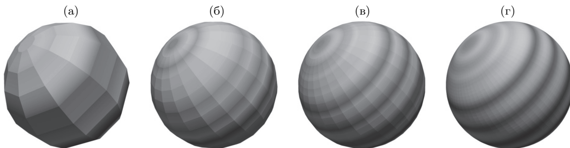
Рис. 2. Сходимость функции плотности \phi(x) .
