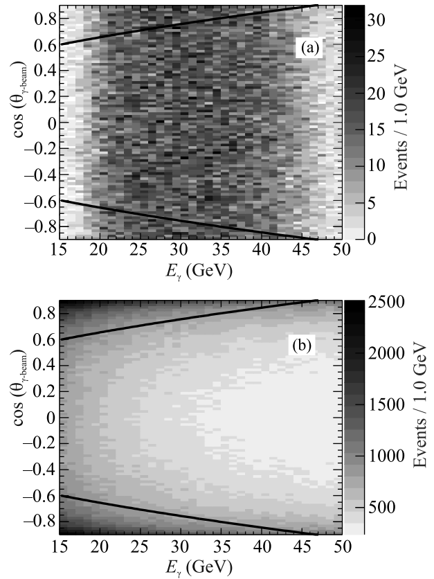
Рис. 3. Двумерные распределения \cos\theta_{\gamma\text{-beam}} в зависимости от E_\gamma для сигнала (а) и суммы значимых фонов (б). Кривые показывают отбор, пояснение к которому дано в тексте
