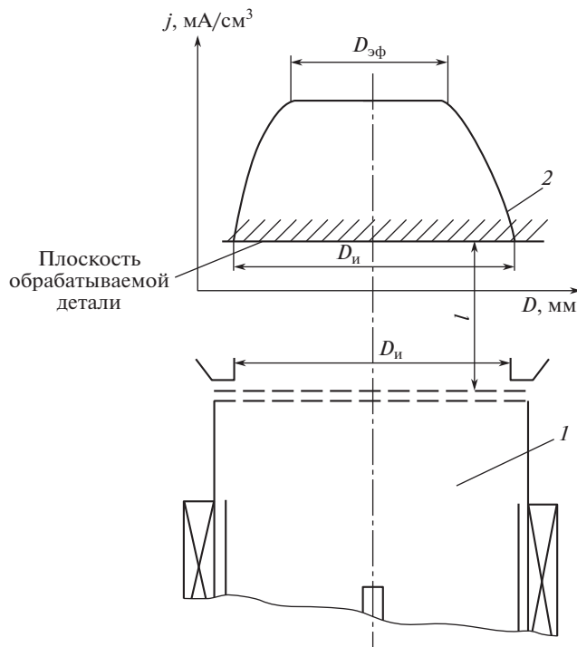
Рис. 3. Распределение плотности ионного тока.
