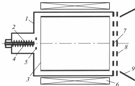
Рис. 2. Принципиальная схема ионного газового источника МАИ-208-2Т.
