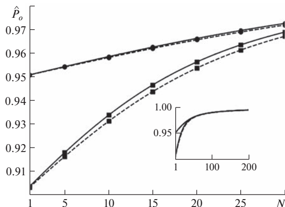
Рис. 5. Сравнение точечных апостериорных оценок вероятности безотказной работы \hat{P}_o , полученных с использованием метода моментов и метода Байеса: сплошная линия — метод моментов; пунктирная линия — метод Байеса. Отметки “квадратом” соответствуют P_b = 0.8 ; “точками” — P_b = 0.9 .
