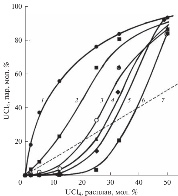
Рис. 3. Изменение концентрации UCl_4 в насыщенных парах его растворов в расплавленных LiCl (1), NaCl (2), NaCl–KCl, 1 : 1 (3), KCl (4), RbCl (5) и CsCl (6) при 1100 К; 7 — изотерма с одинаковыми концентрациями жидкой и паровой фаз.
