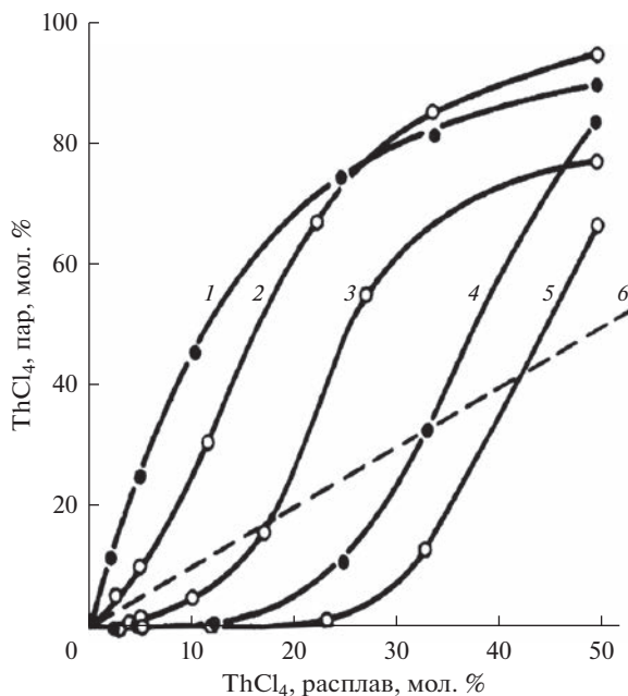
Рис. 4. Изменение концентрации \text{ThCl}_4 в насыщенных парах его растворов в расплавленных \text{LiCl} (1), \text{NaCl} (2), \text{KCl} (3), \text{RbCl} (4) и \text{CsCl} (5) при 1100 К; 6 — изотерма с одинаковыми концентрациями жидкой и паровой фаз.
