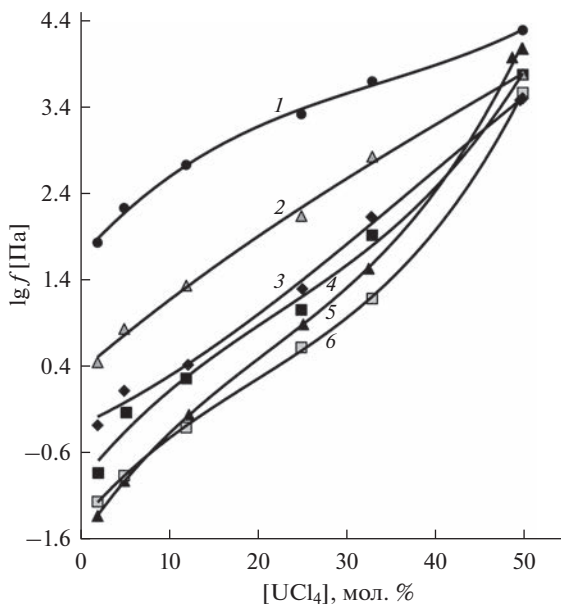
Рис. 2. Изотермы летучести тетрахлорида урана из расплавленных смесей: 1 – \text{UCl}_4\text{--LiCl} , 2 – \text{UCl}_4\text{--NaCl} , 3 – \text{UCl}_4\text{--(NaCl--KCl, 1 : 1)} , 4 – \text{UCl}_4\text{--KCl} , 5 – \text{UCl}_4\text{--RbCl} , 6 – \text{UCl}_4\text{--CsCl} при 1073 К.
