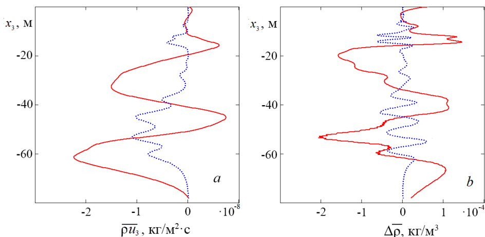
Р и с. 8. Вертикальное распределение волновых потоков массы (a) и генерируемой тонкой структуры (b) для внутренней волны второй моды в горизонтально-неоднородном (красная кривая) и однородном (синяя кривая) случае
