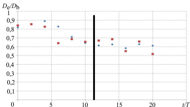
Рис. 7. Зависимость D_e/D_b от t/T . Синие ромбы – эксперимент над конусом с гладкой поверхностью, красные квадраты – эксперимент над конусом с выступом в виде хребта; толстая черная линия – момент времени, когда фронт вихревого течения проходит над хребтом 3 . Соленость воды в бассейне S = 2 \text{ ‰}
