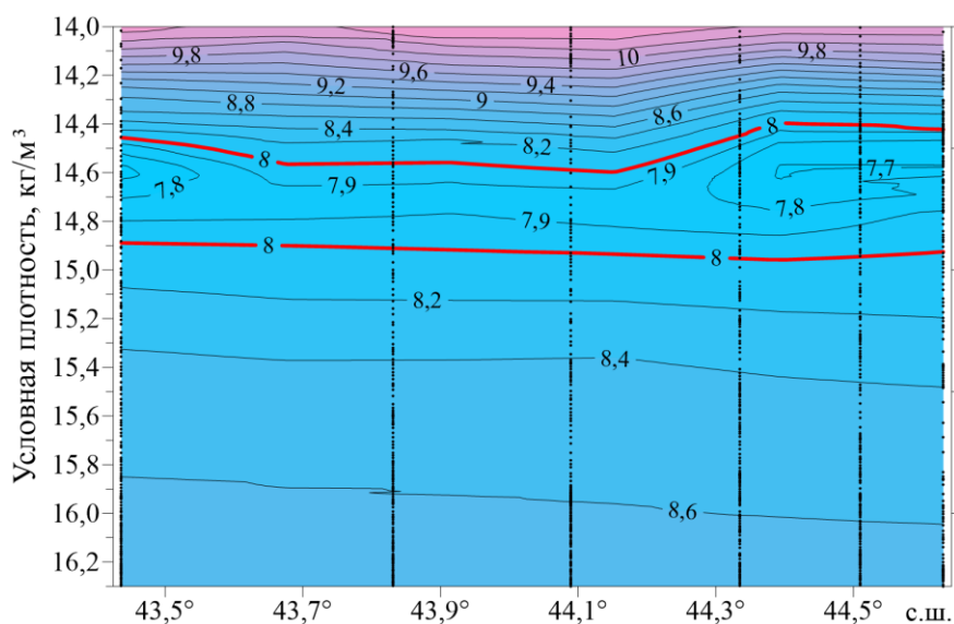
Р и с. 7. Температура на разрезе III в декабре 2017 г. по датчику температуры
