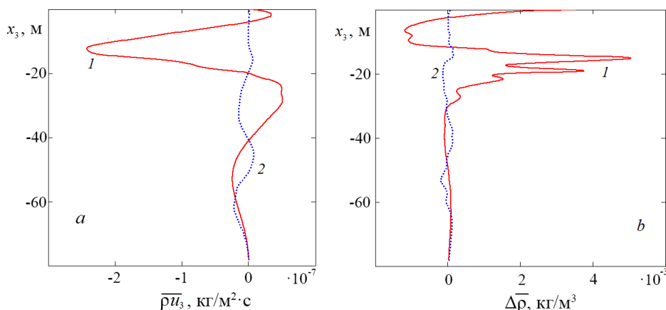
Р и с. 5. Профили вертикального волнового потока массы (a) и тонкой структуры поля плотности (b) для первой (1) и второй (2) мод внутренних волн
