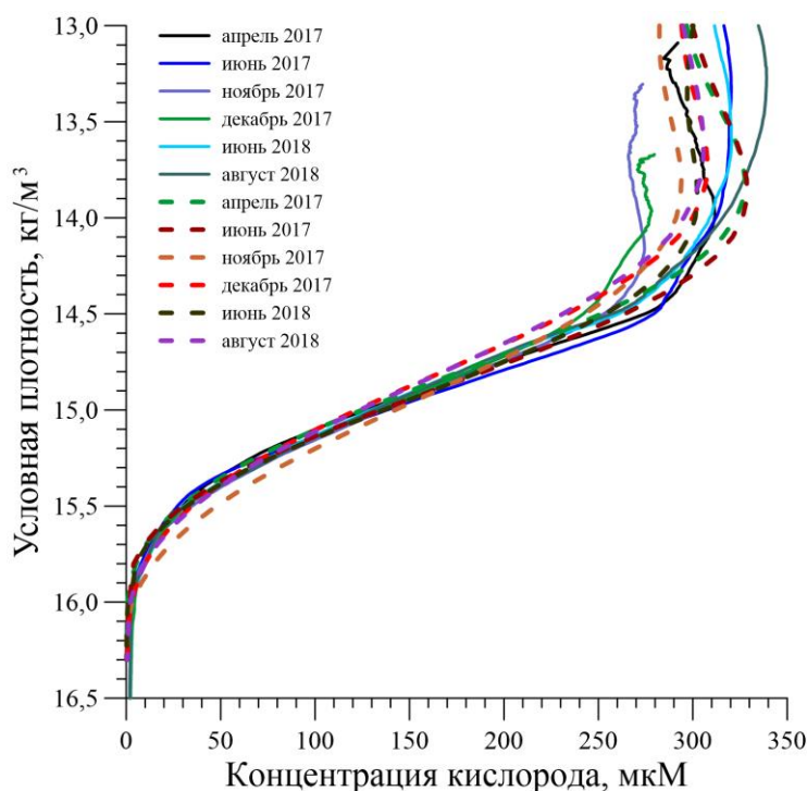
Р и с. 2. Вертикальные профили кислорода в шкале плотности для шести съемок, полученные осреднением данных по методу Винклера (штриховые линии) и по датчику кислорода (сплошные)
