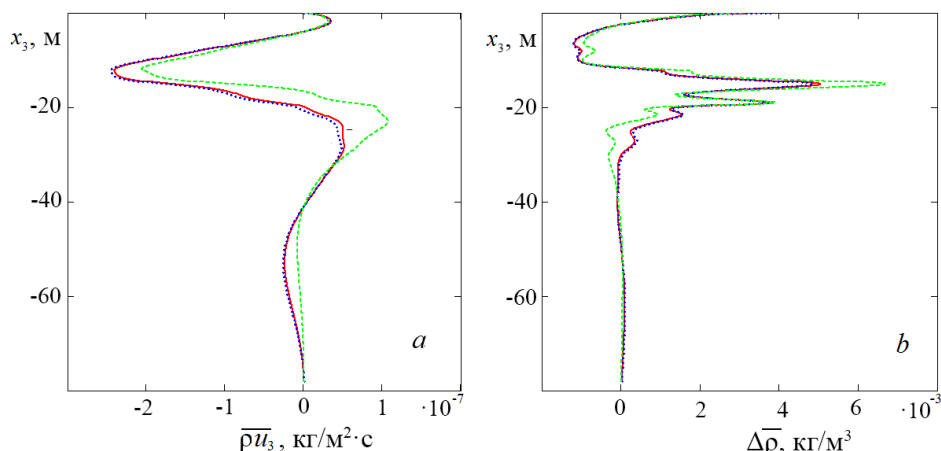
Р и с. 7. Профили вертикального волнового потока массы (а) и тонкой структуры поля плотности (б) у первой моды для 15-минутных внутренних волн (красная кривая), одночасовых внутренних волн (синяя кривая) и 5-минутных внутренних волн (зеленая кривая)
