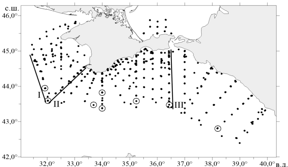
Рис. 1. Схема глубоководных станций, на которых отбирались пробы на кислород и сероводород в 2017–2019 гг. Сплошными линиями обозначены три разреза I – III, которые по возможности выполнялись в каждом рейсе. Кружочками отмечены станции, на которых пробы были отобраны с 37 горизонтов
