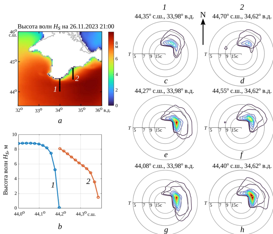
Рис. 7. Затенение волн Крымским п-овом: a – разрезы 1 и 2, наложенные на рассчитанное поле высот волн; b – высота волн вдоль разрезов 1 и 2; частотно-угловые спектры волн вдоль разрезов 1 ( с, е, г ) и 2 ( д, ф, h ), где окружности (от большего к меньшему радиусу) соответствуют периодам волн 5, 7, 9, 15 с Fig. 7. Shading of waves by the Crimean Peninsula: a – transects 1 and 2 superimposed on the simulated field of wave heights; b – wave height along transects 1 and 2; frequency-angular spectra of waves along transects 1 ( c, e, g ) and 2 ( d, f, h ), where the circles (from larger radius to smaller one) correspond to wave periods 5, 7, 9, 15 s
