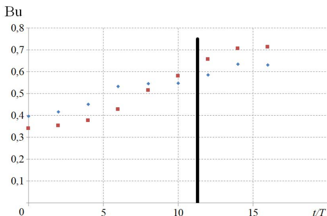
Рис. 8. Зависимость числа Bu от безразмерного времени t/T для S = 2 \text{ ‰}
