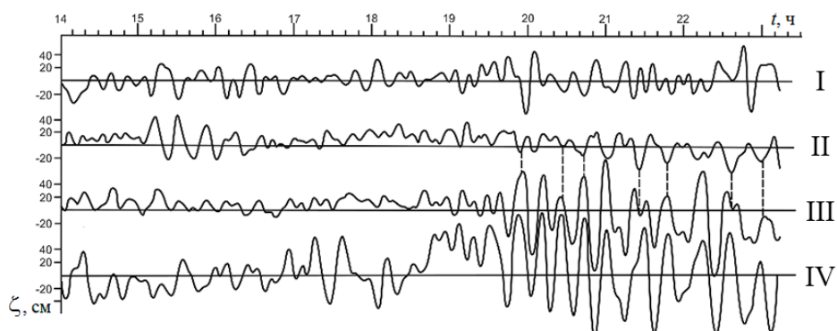
Р и с. 1. Зависимость вертикальных смещений изолиний температуры от времени
