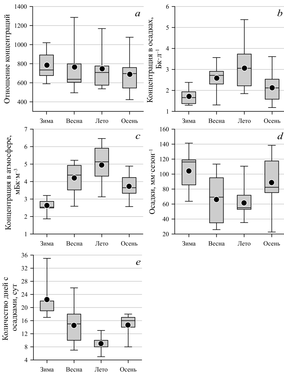
Р и с. 3. Усредненные за весь период наблюдений данные о сезонной изменчивости: отношения концентраций ( a ); концентрации ^7\text{Be} в осадках ( b ); концентрации ^7\text{Be} в атмосфере ( c ); количества осадков ( d ); частоты выпадения осадков ( e )
