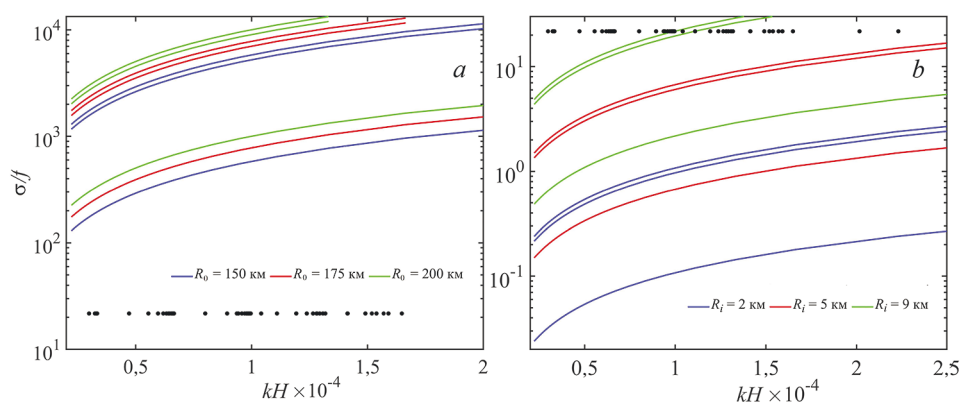
Р и с. 4. Сравнение рассчитанных по альтиметрии характеристик годовых колебаний уровня Балтийского моря (черные точки) с теоретическими дисперсионными кривыми баротропных ( a ) и бароклинных ( b ) топографических волн Россби (линии)
