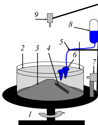
Р и с. 2. Схема экспериментальной установки 2,3 : 1 – циклонически вращающаяся платформа; 2 – цилиндрический бассейн из оргстекла; 3 – конус; 4 – выступ в виде хребта; 5 – трубка; 6 – вытекающая из источника подкрашенная вода и образующиеся под ним антициклонические вихри; 7 – видеокамера сбоку; 8 – объемная бюретка с краном; 9 – видеокамера сверху
