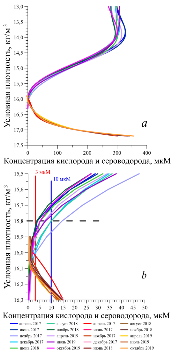
Р и с. 3. Вертикальные профили кислорода и сероводорода в Черном море в 2017–2019 гг. в шкале плотности во всей толще (a) и более подробно – в интервале \sigma_t = 15,5-16,3 \text{ кг/м}^3 (b) F i g. 3. Vertical profiles of oxygen and hydrogen sulfide in the density scale over the entire thickness (a) and in the interval \sigma_t = 15,5-16,3 \text{ kg/m}^3 (b) in the Black Sea in 2017–2019
