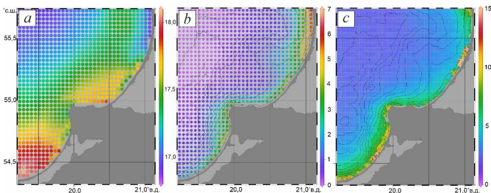
Р и с. 2. Средние за летний сезон 2000–2019 гг.: значения ТПМ ( ^\circ\text{C} ) – a , повторяемость апвеллингов (среднеголетнее количество дней с отрицательной температурной аномалией за месяц или за сезон в заданной ячейке) – b и концентрация хлорофилла a (до 15\text{ mg/m}^3 ) – c Fig. 2. Summer season mean values of SST ( ^\circ\text{C} ) – a , upwelling repeatability (multi-year average number of the days with negative temperature anomaly per month or season in a given cell) – b , and Chl a concentration (up to 15\text{ mg/m}^3 ) – c in 2000–2019
