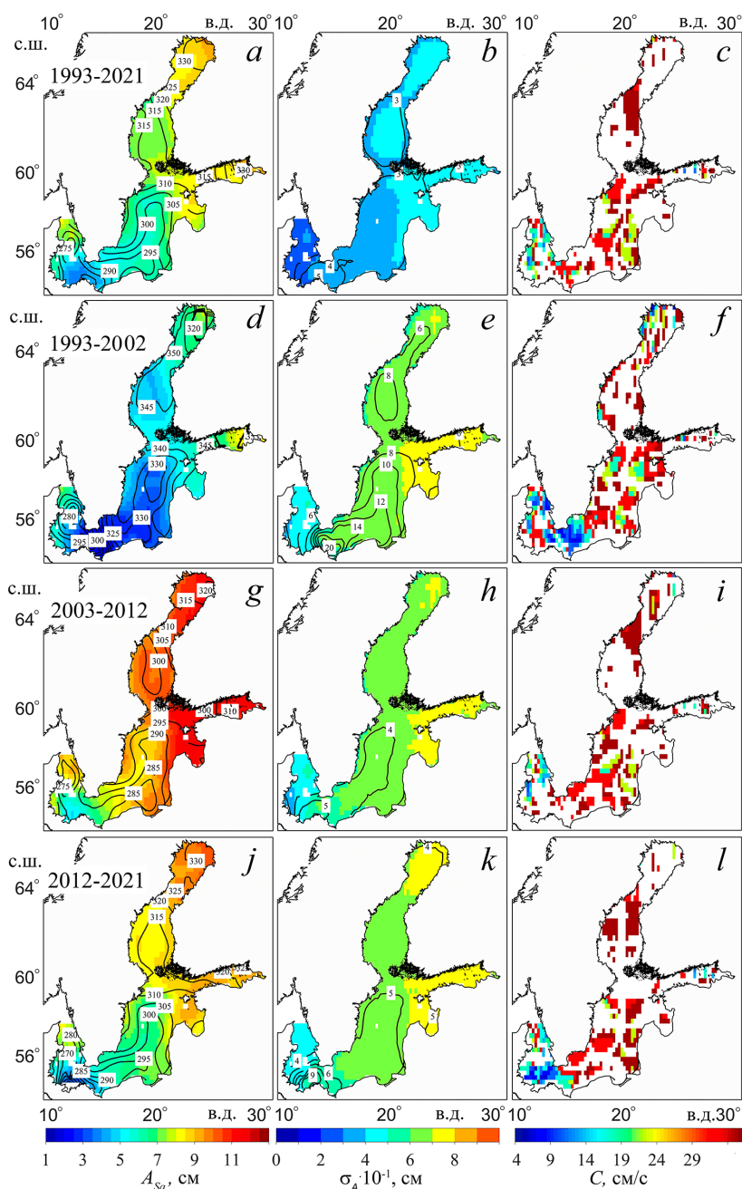
Р и с. 2. Амплитудно-фазовые характеристики годовой гармоник S_a в Балтийском море, оцененные по данным спутниковой альтиметрии (изолиниями обозначены фазы в градусах) ( a, d, g, j ), среднеквадратические ошибки оценок амплитуды и фазы (изолинии) годовой гармоник ( b, e, h, k ) и оценки скорости перемещения годовых колебаний уровня моря, рассчитанные по формуле (1) ( c, f, i, l ), за 1993–2021 ( a – c ), 1993–2002 ( d – f ), 2003–2012 ( g – i ) и 2012–2021 гг. ( j – l ) F i g. 2. Amplitude-phase characteristics of annual harmonic S_a in the Baltic Sea assessed by satellite altimetry data (isolines indicate phases in degrees) ( a, d, g, j ), root-mean-square errors in the estimates of amplitude and phase (isolines) of the annual harmonic ( b, e, h, k ), and estimates of motion velocity of annual fluctuations of sea level calculated by formula (1) ( c, f, i, l ) for 1993–2021 ( a – c ), 1993–2002 ( d – f ), 2003–2012 ( g – i ) and 2012–2021 ( j – l )
