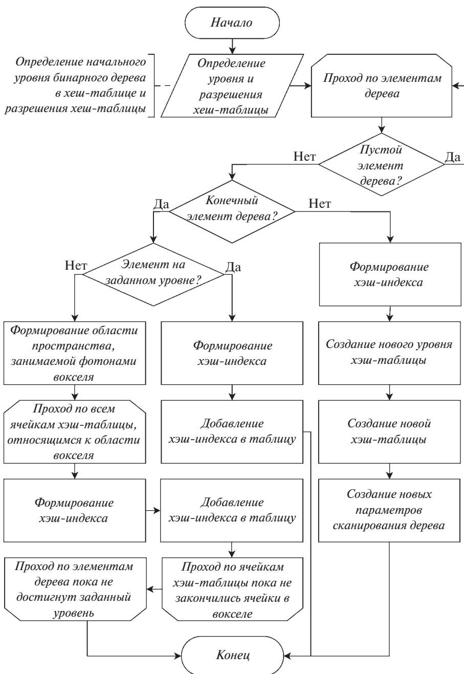
Рис. 4. Алгоритм построения хеш-таблиц.
