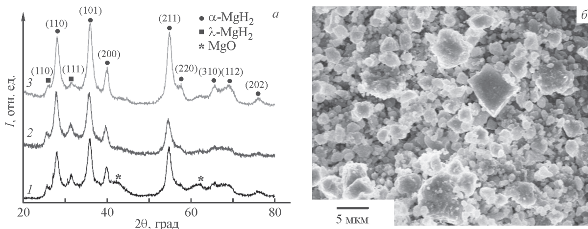
Рис. 1. Дифрактограммы: 1 — MgH 2 , 2 — композита MgH 2 с графеноподобным материалом, 3 — композита MgH 2 с никель-графеновым материалом (а); микрофотография композита MgH 2 с никель-графеновым материалом, полученная с помощью сканирующего электронного микроскопа (б).
