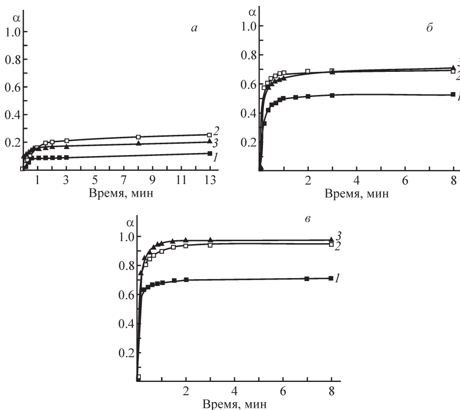
Рис. 2. Зависимость степени превращения от времени в реакции MgH 2 (1), композитов MgH 2 с графеноподобным (2) и никель-графеновым материалами (3) с водой (а), 0.1 М (б) и 0.3 М (в) раствором лимонной кислоты.
