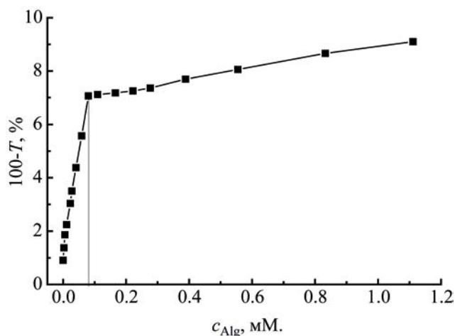
Рис. 2. Зависимость мутности смешанной системы VR–Alg от концентрации Alg при фиксированной концентрации VR 0.01 mM. в воде ( \lambda 450 nm, l 10 mm, 25°C).
