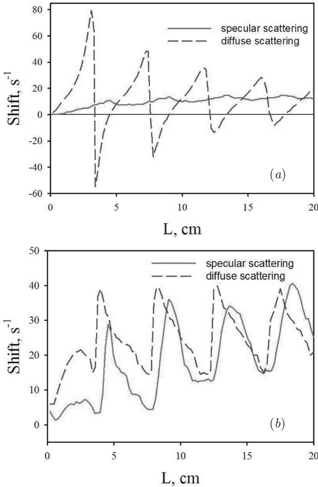
Рис. 3. Сдвиги положения абсолютного максимума контраста резонанса КПН в зависимости от размеров ячейки для двух типов отражения — зеркально-когерентного и диффузного. Расчеты проведены для следующих параметров: \Omega_1 = \Omega_2 = 3 \cdot 10^5 \text{ с}^{-1} ; \lambda_{hfs} = 4.5 \text{ см} ; T = 50^\circ \text{C} ; \Delta_1 = \Delta_2 = 0 ; \omega_{34} = 800 \text{ МГц} (a); \omega_{34} = 400 \text{ МГц} (b). Остальные параметры те же, как на рис. 2. Покрытие идеальное ( \alpha = 1, \beta = 1 )
