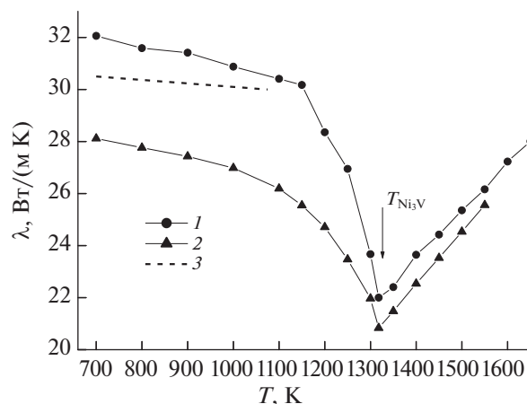
Рис. 4. Политермы коэффициента теплопроводности сплава Ni–25 ат. % V: 1 — полная теплопроводность, 2 — электронная составляющая, 3 — данные [28].
