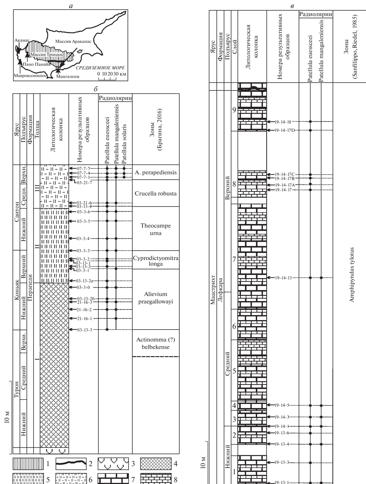
Рис. 1. Местонахождение изученных радиолярий на Кипре ( а – схема); б, в – литологические колонки: б – композитный разрез Мангалени (формация Перапеди, турон–сантон), в – разрез Пано Панайя (формация Лефкара, маастрихт). Обозначения: 1 – офиолитовый массив Троодос; 2 – разлом Аракапас; 3 – верхние пиллоу-лавы; 4 – умбри-ты с прослоями радиоляриевых кремней и массивных абиогенных кремней; 5 – кремни с прослоями кремнистых ар-гиллитов; 6 – кремни опоквидные, марганцовистые; 7 – известняки; 8 – мергели.
