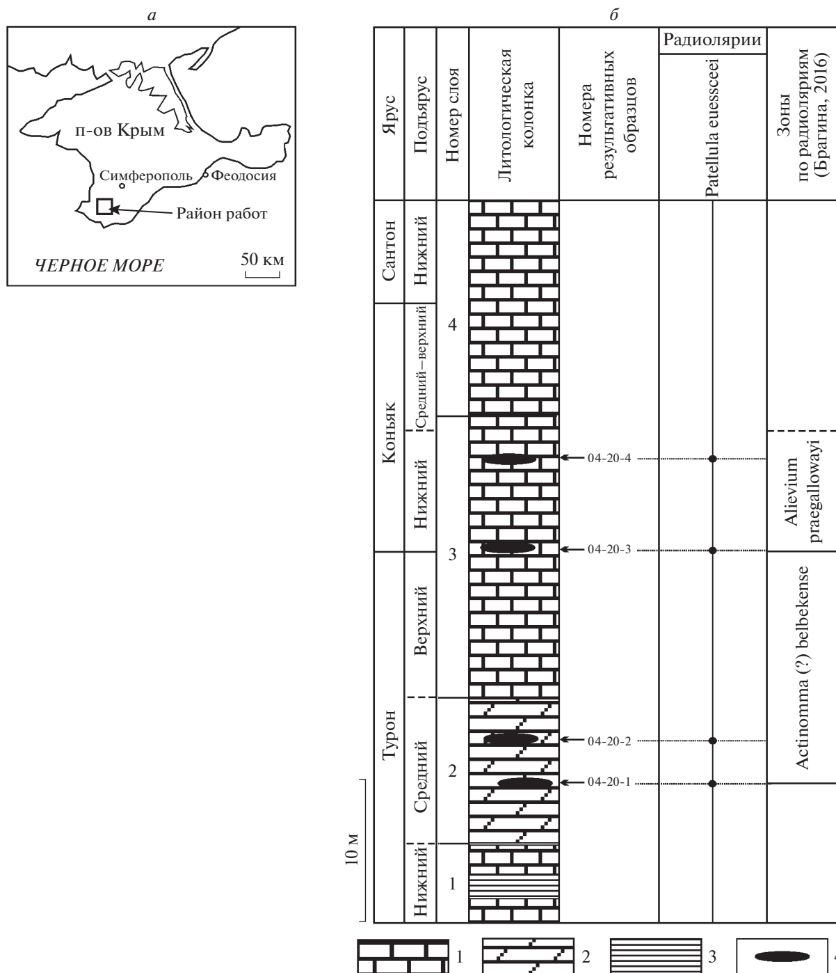
Рис. 3. Местонахождение изученных радиоларий в юго-западной части Горного Крыма: a — схема; б — литологическая колонка отложений турона—сантона горы Чуку (по: Брагина, 2014, рис. 1, г ; с дополнением по: Брагина, 2016). Обозначения: 1 — известняки, 2 — мергели; 3 — глины; 4 — стяжения кремней.
