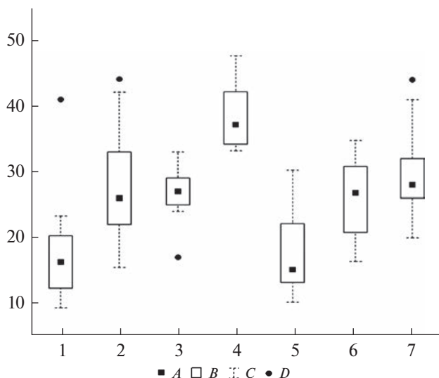
Рис. 3. Видовая насыщенность растительности хвойно-широколиственных лесов р. Пшехи. Примечание. По оси абсцисс — типы леса (1 — пихто-буковые папоротниково-разнотравные; 2 — пихто-грабовые оино-разнотравные; 3 — осино-грабовые жимолостно-мелкотравные; 4 — грабово-черноольховые нитрофильно-высокотравные; 5 — грабово-дубовые рододендро-ожиновые; 6 — грабово-буковые оино-разнотравные; 7 — грабовые жимолостно-ожиновые); по оси ординат — число видов: A — медианы, B — диапазоны между квантилями, C — диапазоны между минимумом и максимумом, D — выбросы.
