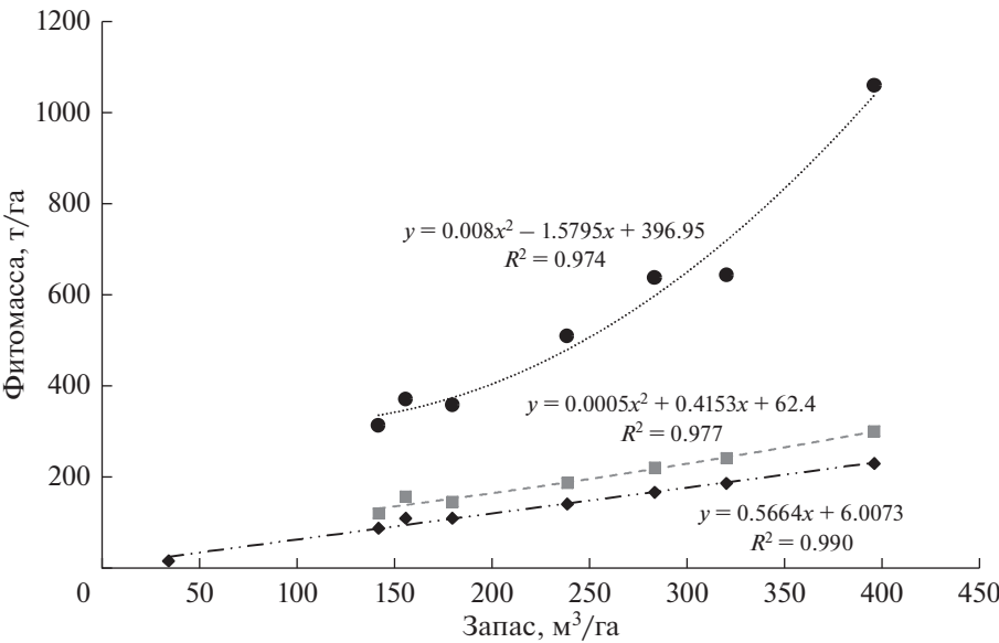
Рис. 2. Зависимость между общей продуктивностью ( P_{\text{общ}} ●), фитомассой лиственных насаждений ( P_{\text{л}} ■) и древостоев ( P_{\text{д}} ◆) и запасом.
