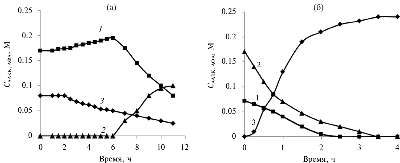
Рис. 4. Гидрирование изомеров \alpha\text{-AAKK}_1 (1) и \alpha\text{-AAKK}_2 (2) на каталитической системе \text{Pd}(\text{Asac})_2\text{-I-H}_2 с образованием N\text{-АФА} (3) (а) T = 25^\circ\text{C} ; б) T = 60^\circ\text{C} ; P_{\text{H}_2} = 5 Бар, растворитель – смесь толуол : метанол = 3 : 17).
