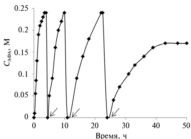
Рис. 6. Образование N-АФА на системе \text{Pd}(\text{Acac})_2 -Cin- \text{H}_2 ( C_{\text{Pd}} = 0.31 мМ; Sub/Pd = 1000; V_{\text{p-ра}} = 20 мл, T = 60^\circ\text{C} ; P_{\text{H}_2} = 5 атм, стрелками указано время внесения порции субстрата).
