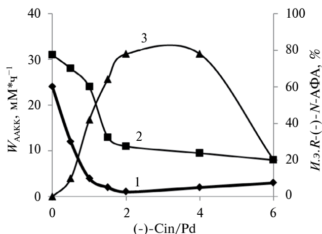
Рис. 5. Зависимость скорости гидрирования изомеров \alpha -ААКК 2 (1), ААКК 1 (2) и и.э. (R)-(-)-N-АФА (3), на каталитических системах \text{Pd}(\text{Acac})_2 - n Cin- \text{H}_2 от мольного отношения 1/Pd.
