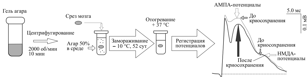
Рис. 1. Схема протокола приготовления замораживающей среды с легкой фракцией агара и регистрация АМПА- и НМДА-потенциалов после криосохранения.
