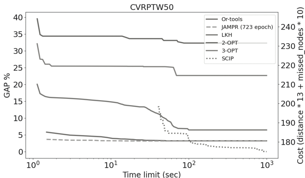
Рис. 4. Эффективность моделей на CVRPTW с 50 точками.
