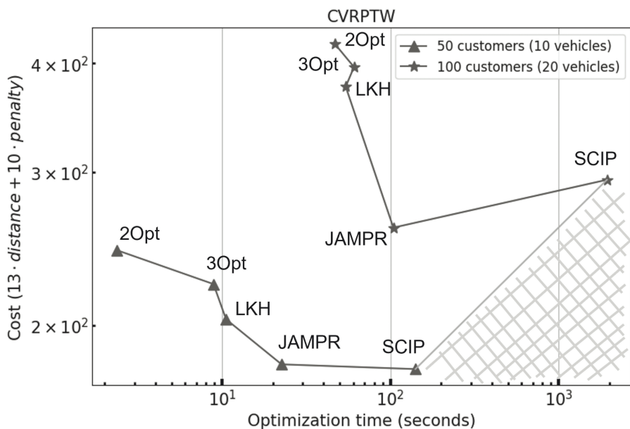
Рис. 3. Итоговый результат классических подходов.
