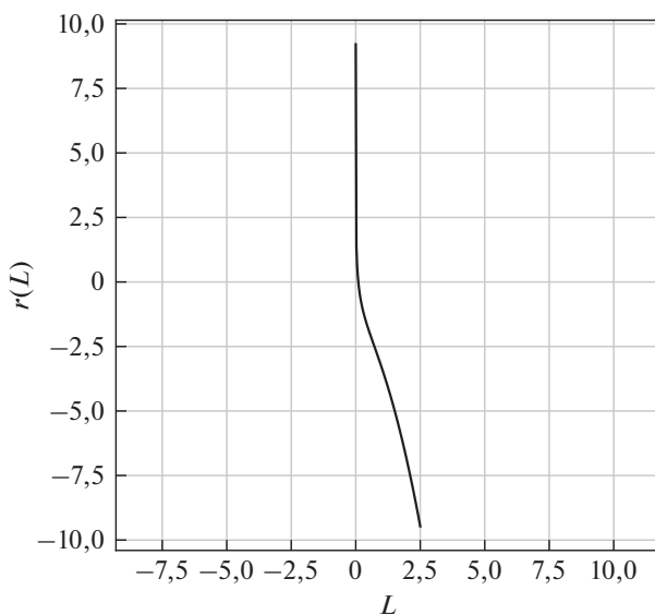
Рис. 6. График зависимости вознаграждения от расстояния между агентами.
