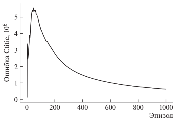
Рис. 9. Зависимость значения функции ошибки от эпизода сети Critic.
